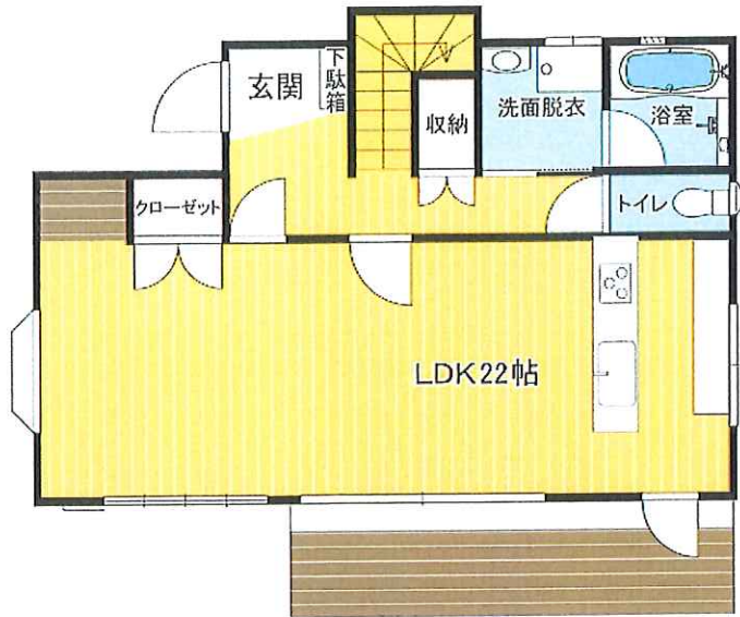
1階 間取図
