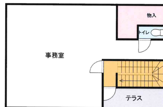
3階 間取図
