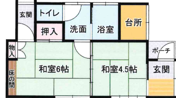
別棟 間取図
